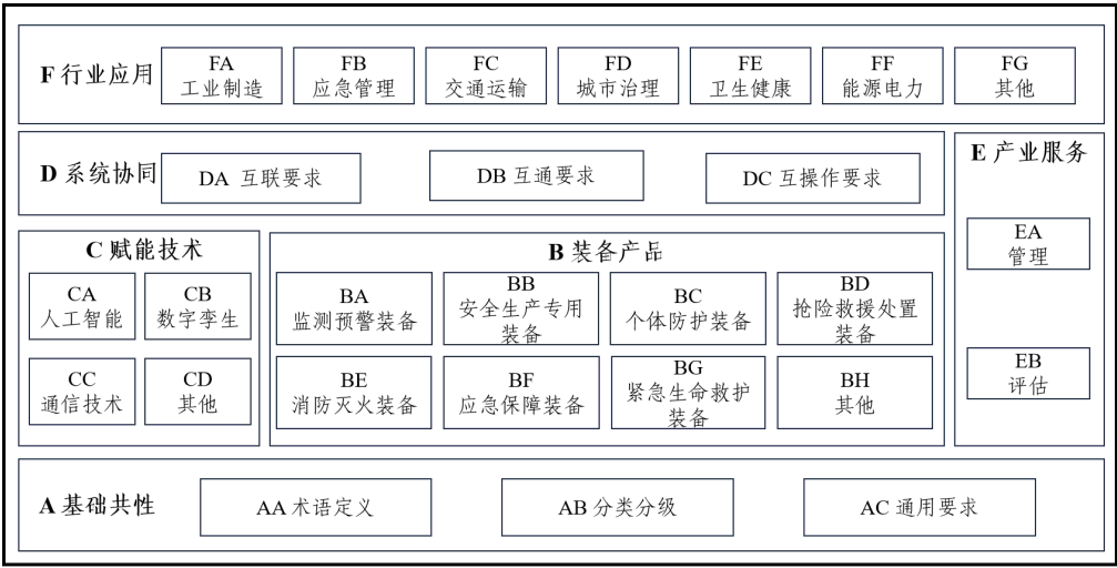
图 1 安全应急装备标准体系结构图
